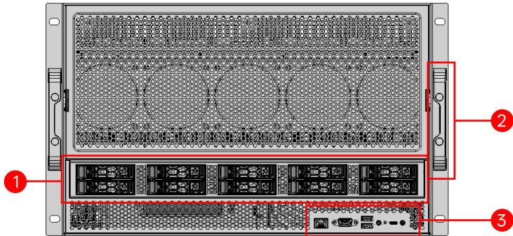
图5-1 前面板视图
