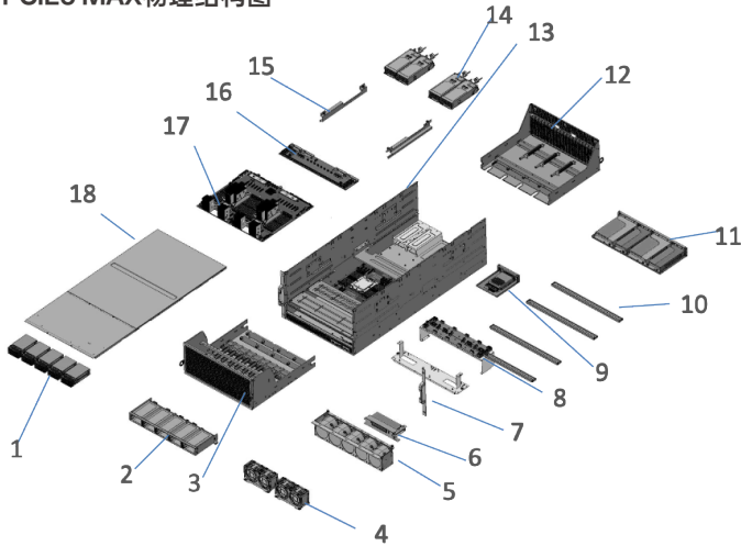
图4 G5208 PCIe5 MAX物理结构图
