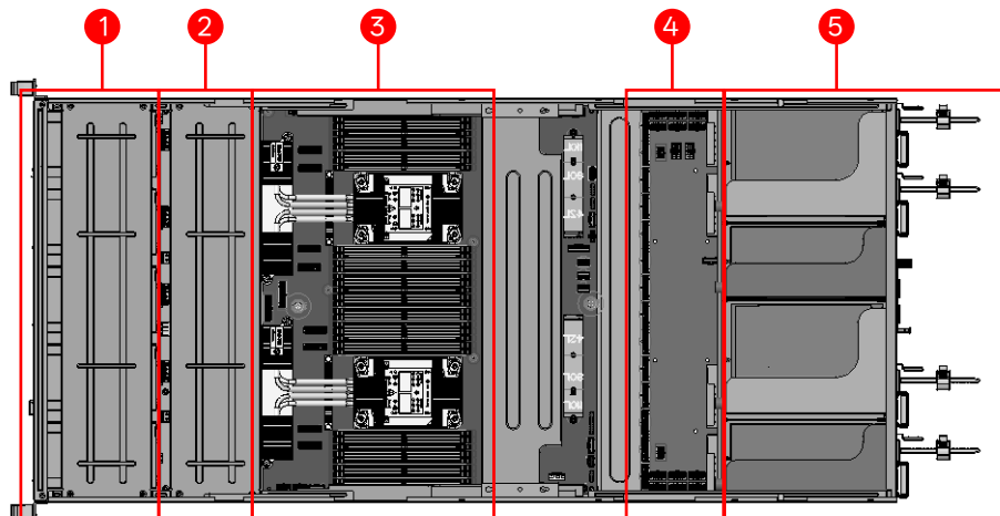
图5-4 内部视图-CPU层
