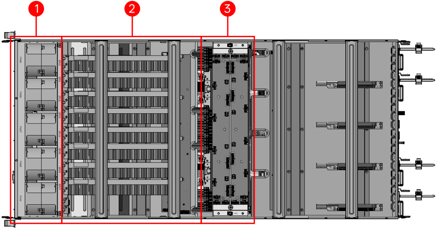
图5-4 内部视图-GPU层
