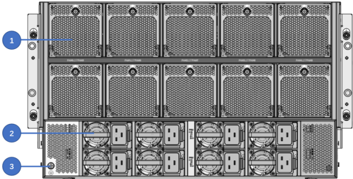
图3-2 后面板视图
