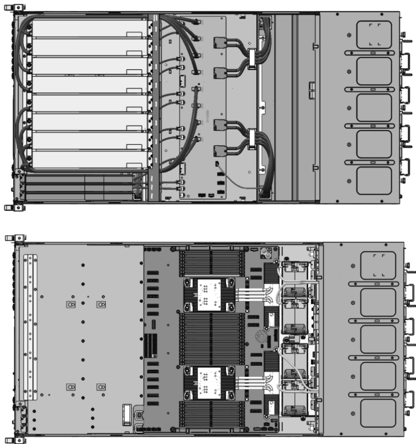
图3-3 内部视图-GPU层
