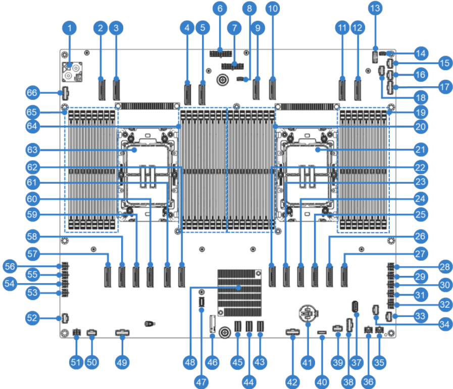
图3-4 主板图布局
