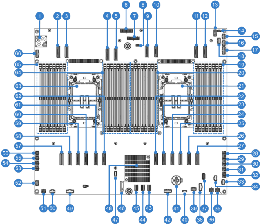
图5-5 主板图布局
