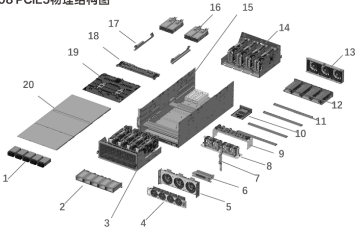
图4 G5208 PCIe5物理结构图
